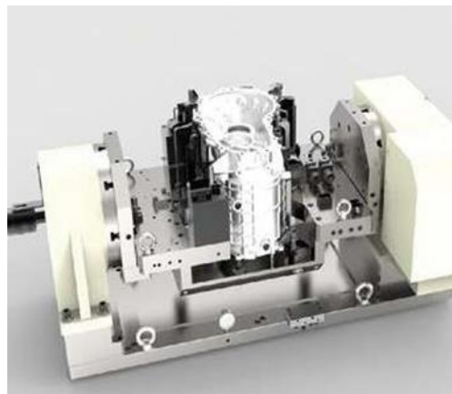
治具 fixture
