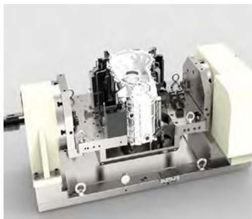
治具 fixture
